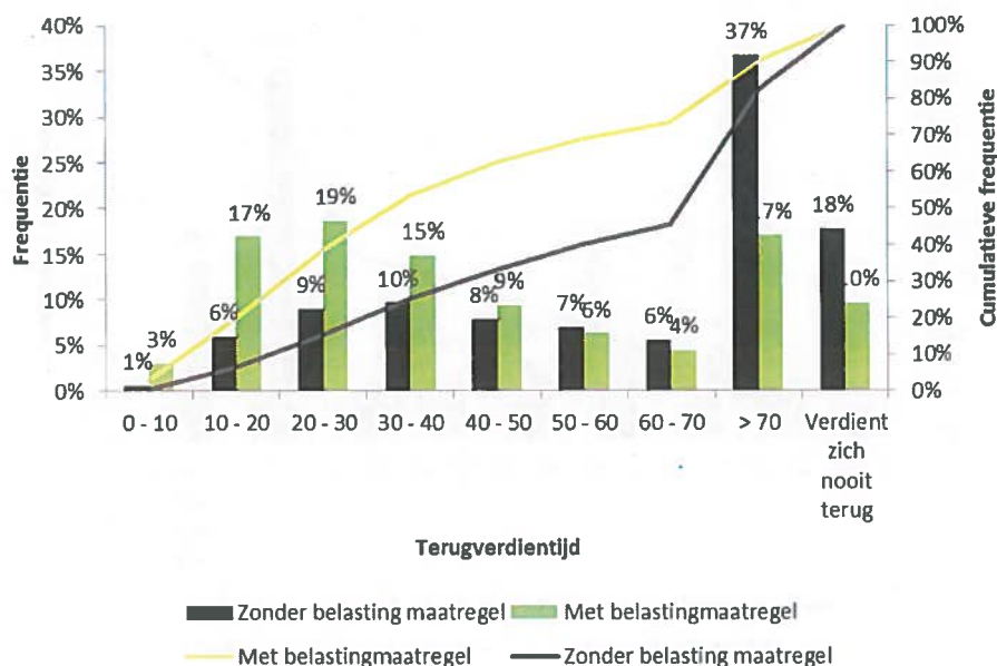
Figuur 4: Effect belastingaanpassing op de terugverdiëntijd van een warmtepomp (zonder extra isolatie), zonder kosten voor rente. Zichtjaar 2020.
