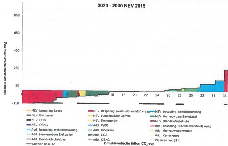
Figuur 23: Kostencurve maatregelen NEV2015 2020-2030 vastgesteld en voorgenomen beleid
