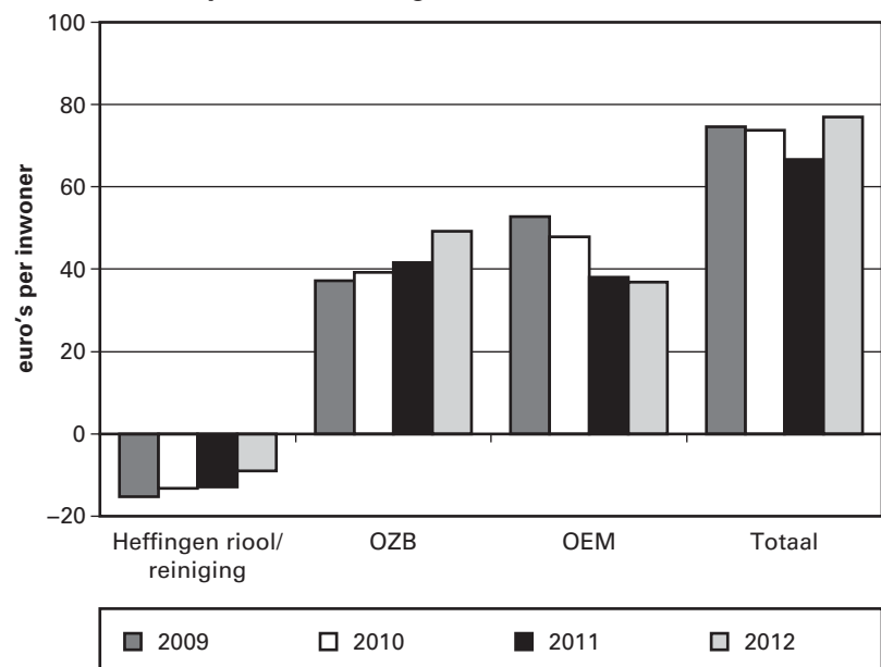
Figuur 3.3. Verschil tussen de feitelijke en veronderstelde netto-inkomsten bij de clusters Riol, Reiniging, OZB en OEM (exclusief de mutatie reserves), 2009 t/m 2012 (euro's per inwoner; 373 gemeenten)
