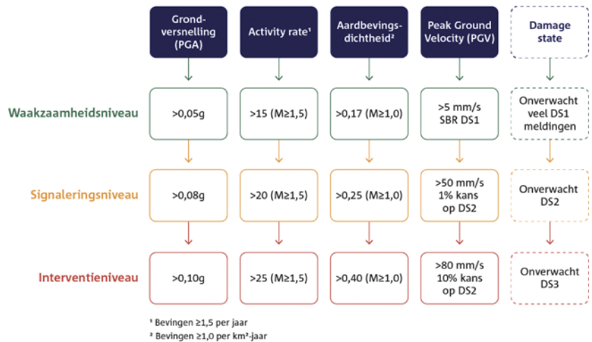
Figuur 6.3 Meet- en regelprotocol voor het Groningenveld
