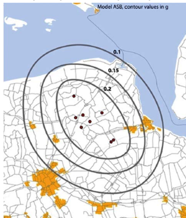
Figuur 5.2 Contouren van de maximale grondversnelling (PGA, in g) bij een aardbeving van magnitude 5,0 in de regio Groningen
