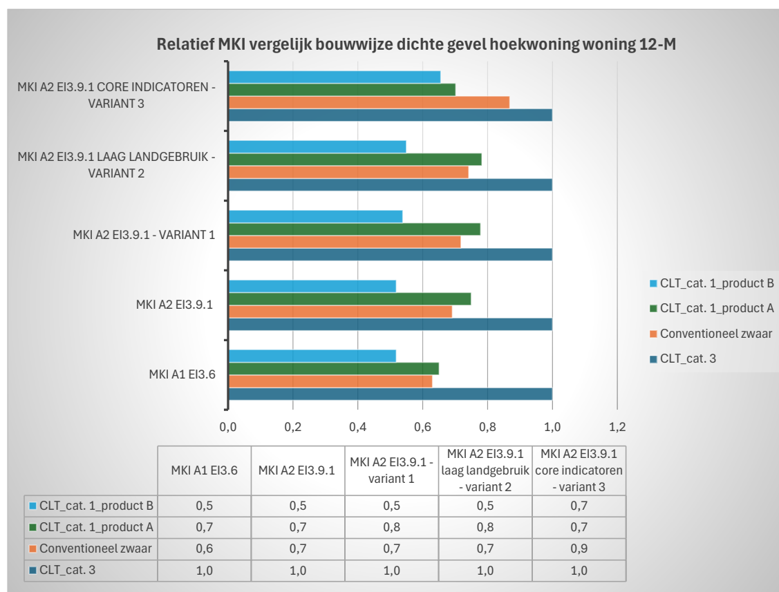
Figuur 9: vergelijking rekenresultaat dichte gevel tussenwoning 13M met categorie 3 CLT als referentie
