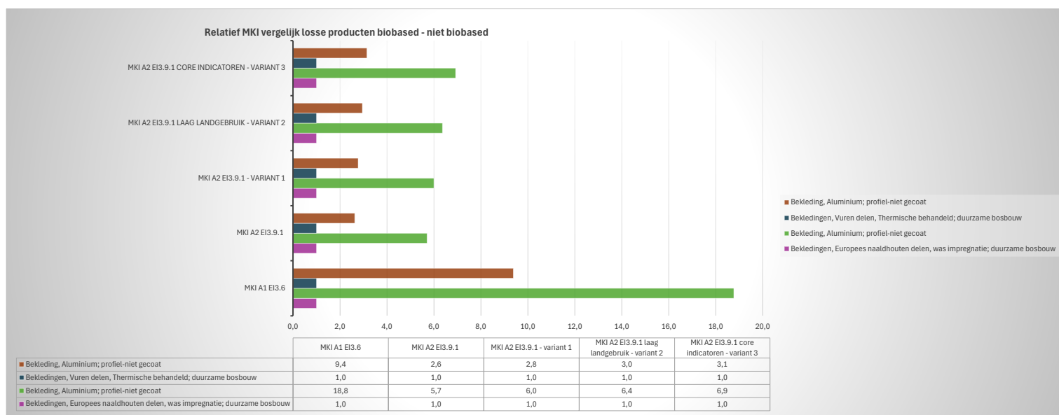
Figuur 16: vergelijking rekenresultaat gevelbekleding
