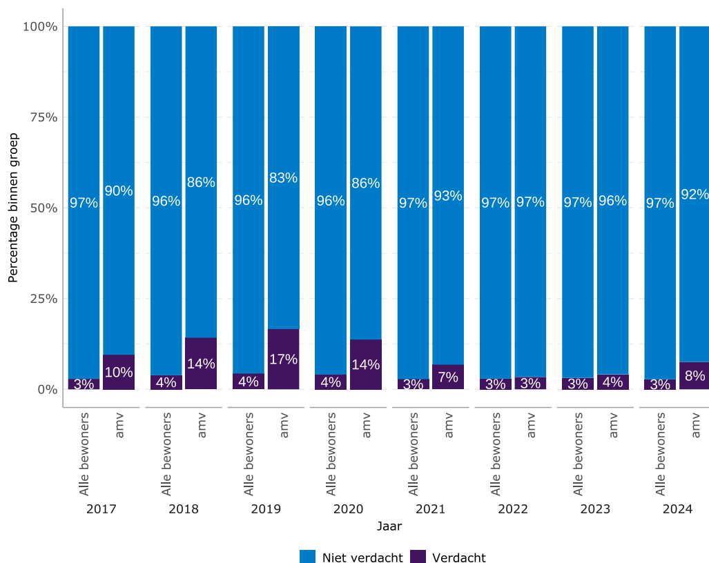
Figuur 4.6 Aandeel verdachten onder totale groep COA-bewoners en onder amv's
