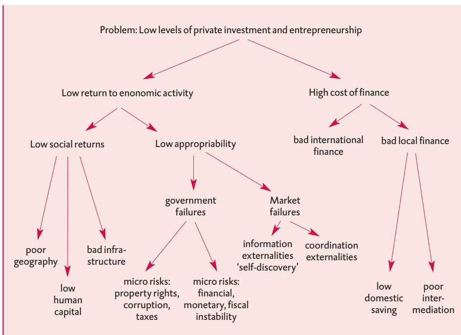
Figuur 7.1 Groeidiagnostiek
