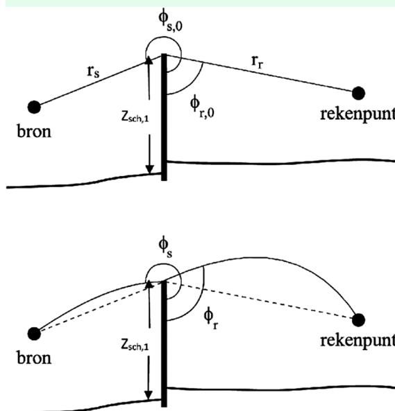
Figuur 4.10: Straalkromming
