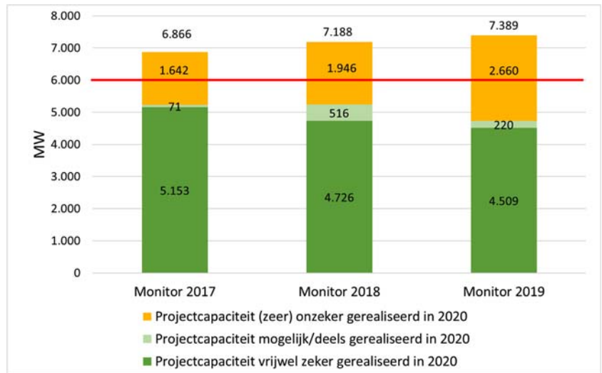
Figuur 1 Inschatting haalbaarheid realisatie in 2020 van de in ontwikkeling zijnde projecten (op basis van de doorgegeven ingebruikname-data door de initiatiefnemers in de Monitor Wind op Land 2019, RVO.nl)
