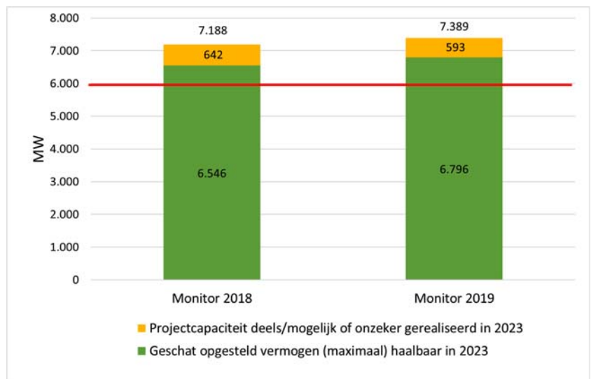
Figuur 2 Inschatting haalbaarheid realisatie in 2023 van de in ontwikkeling zijnde projecten (op basis van de Monitor Wind op Land 2019, RVO.nl)
