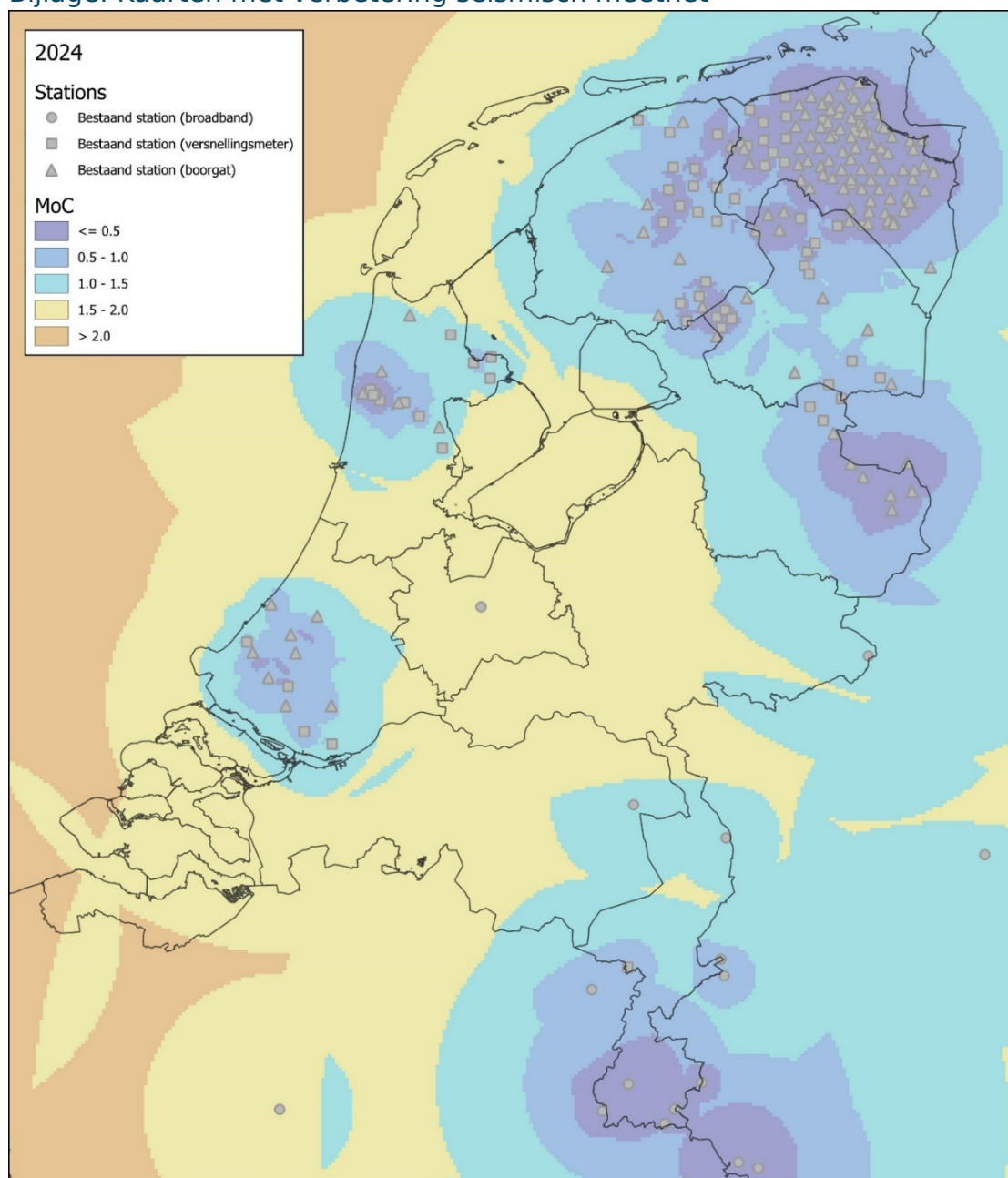
Figuur 1. Magnitude waarboven alle aardbevingen onder gebruikelijke condities gelokaliseerd worden door het meetnet 6 , situatie september 2024.
