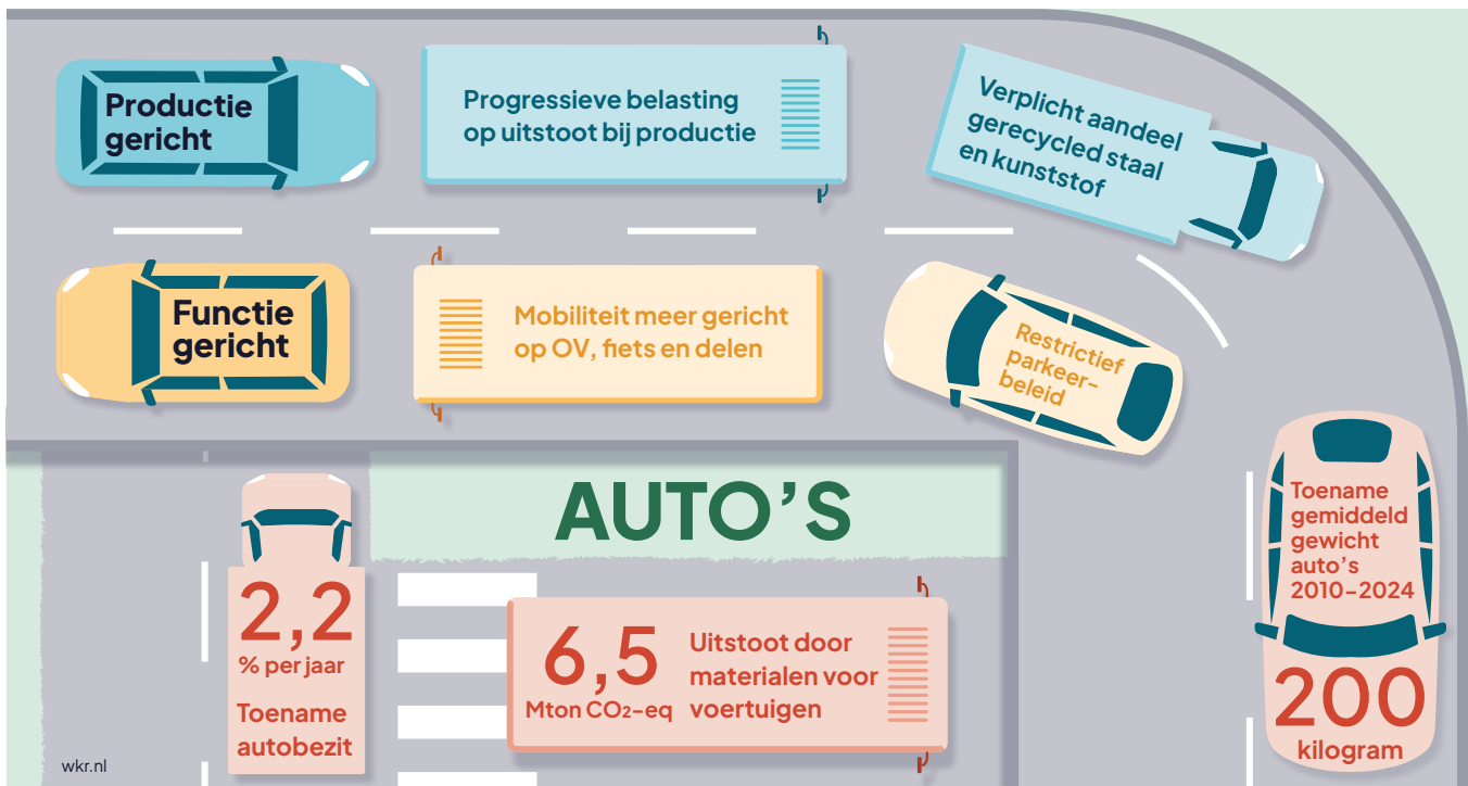
Figuur 10. Bronnen van getallen van links naar rechts): RVO & Revnext (2025), CBS (2025a) en CBS (2025d).
