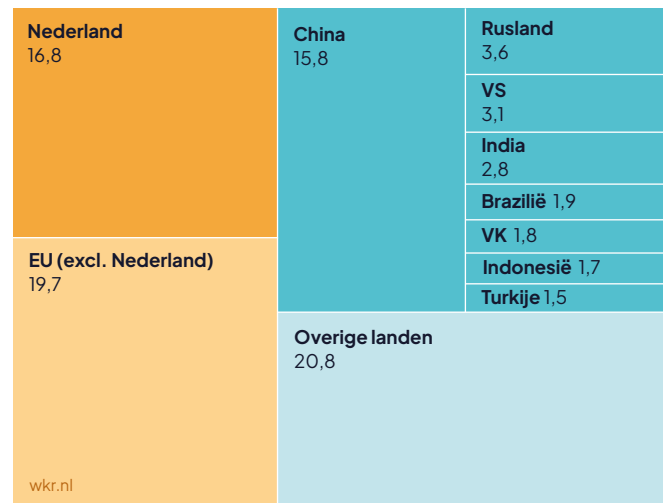
Figuur 4. In de uitsplitsing worden alle landen getoond met een aandeel van minstens 1 MtCO 2 -eq. in de Nederlandse voetafdruk. Eigen analyse op basis van CBS (2025a).
