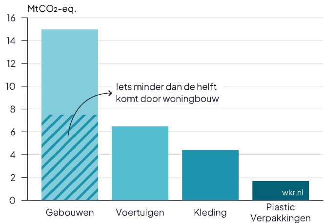
Figuur 9. Data voor gebouwen, voertuigen en kleding volgen uit eigen analyse op basis van CBS (2025a), voor verpakking op basis van RIVM (2024). Aandeel van woningbouw op basis van Rli (2025a), de rest van de uitstoot komt door utiliteitsbouw, zoals kantoren en ziekenhuizen.
