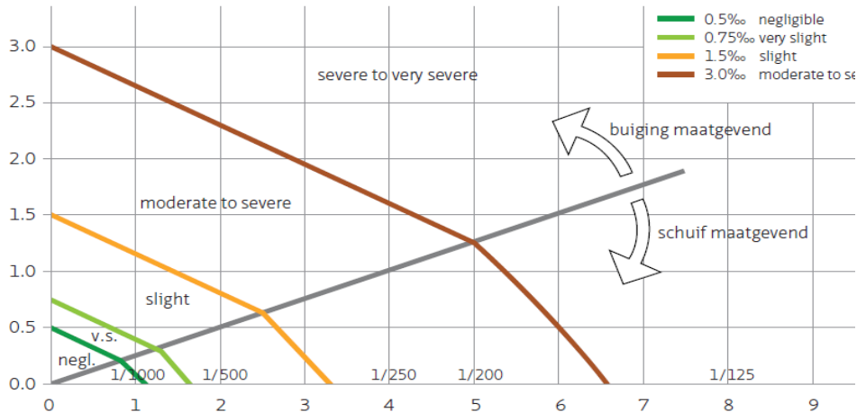
Figuur 12.5 – schadecriteria m.b.t. horizontale rek en hoekvervorming naar Son & Cording [12.11]. Horizontaal staat de hoekvervorming in 10^{-3} en verticaal de horizontale rek in 10^{-3} .
