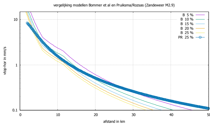
Figuur 7.7: vergelijking van de modellen van Bommer et al (aangeduid met B) en Pruiksm/Rozsas (aangeduid met PR) voor de beving Zandeweer (2014-11-05) met magnitude 2,9.
