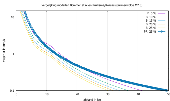
Figuur 7.8: vergelijking van de modellen van Bommer et al (aangeduid met B) en Pruiksm/Rozsas (aangeduid met PR) voor de beving Garmerwolde (2014-09-30) met magnitude 2,8.
