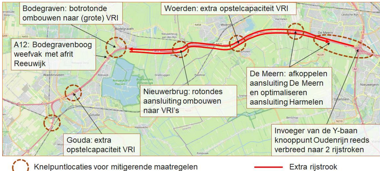
Figuur 2: Overzicht maatregelenpakket 'partiële verbreding A12'
