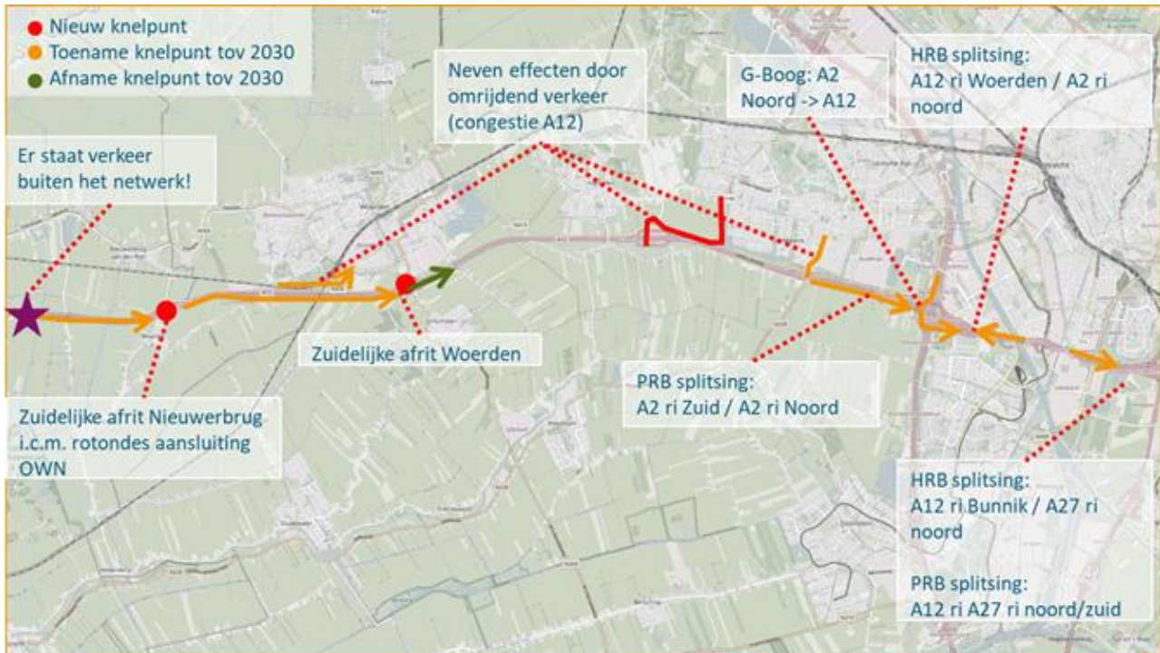
Figuur 16: Knelpunten (Filelocaties) ochtendspits 2030 extra rijstrook t.o.v. 2030 autonome situatie
