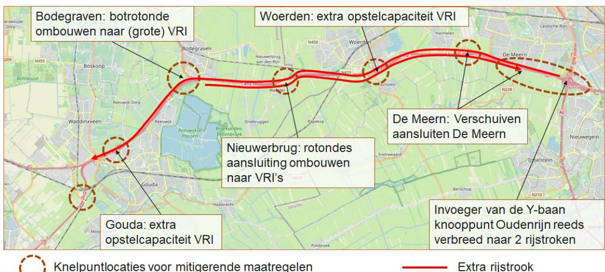
Figuur 3: Overzicht maatregelenpakket 'asymmetrische verbreding A12'
