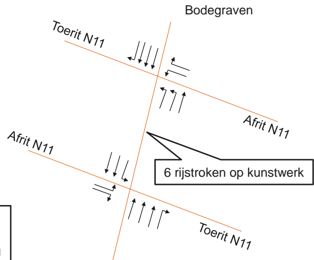
Figuur 32: Aanpassingen Botrotonde Bodegraven in alle drie maatregelpakketten
