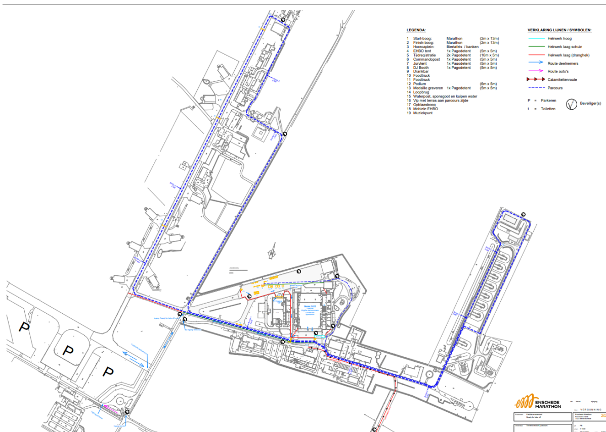
Bijlage 2. Overzicht terrein startgebied
