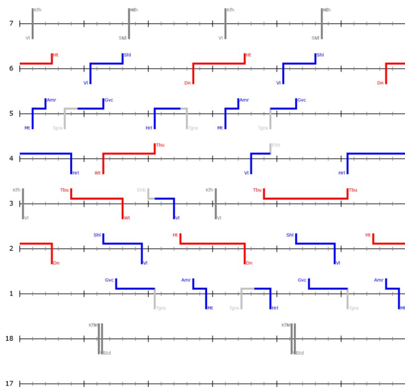
Figuur 10: Spooropstelling Eindhoven MLT 2026 in avonduren optie 1
