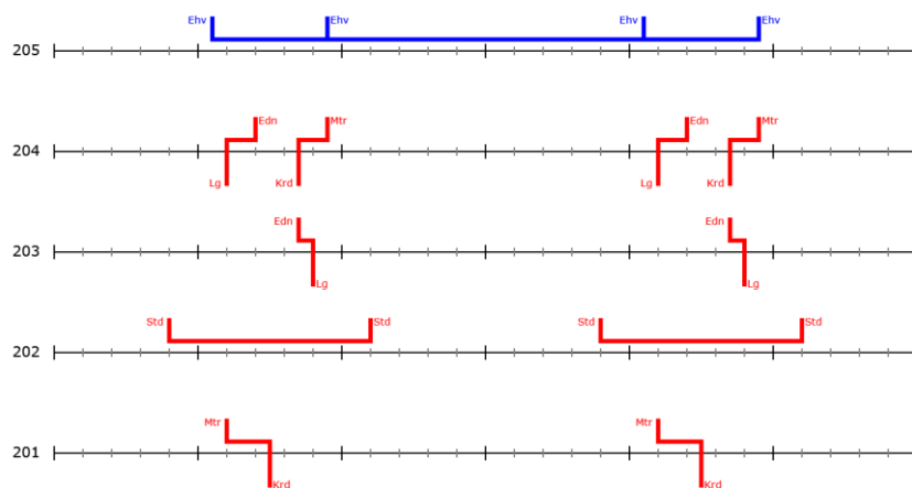
Figuur 11: Spooropstelling Heerlen MLT 2026 in avonduren optie 1
