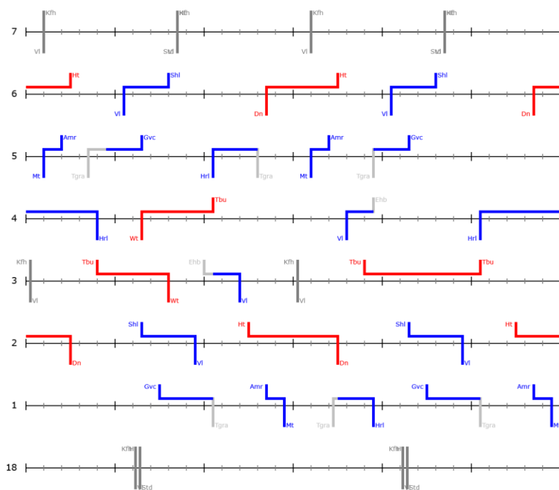
Figuur 18: Spooropstelling Eindhoven MLT 2026 in avonduren optie 2
