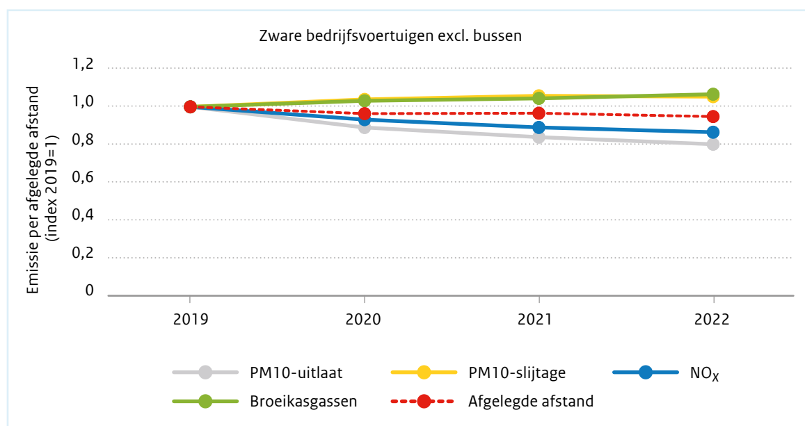
Figuur 4.27 Emissie per afgelegde afstand voor vrachtauto's (inclusief trekkers), 2019-2022. Bronnen: afgelegde afstand: CBS; emissies: Emissieregistratie; bewerking KiM. Het gaat om tank-to-whelemmissies. De uitstoot van broeikasgassen is inclusief de uitstoot door verbranding van biobrandstof.
