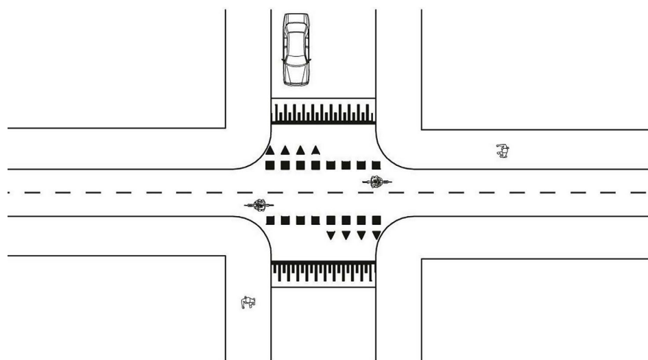
Afbeelding 5.1. Oversteek solitair fietspad met plateau volgens ASVV 14.2.15 (CROW, 2021)
