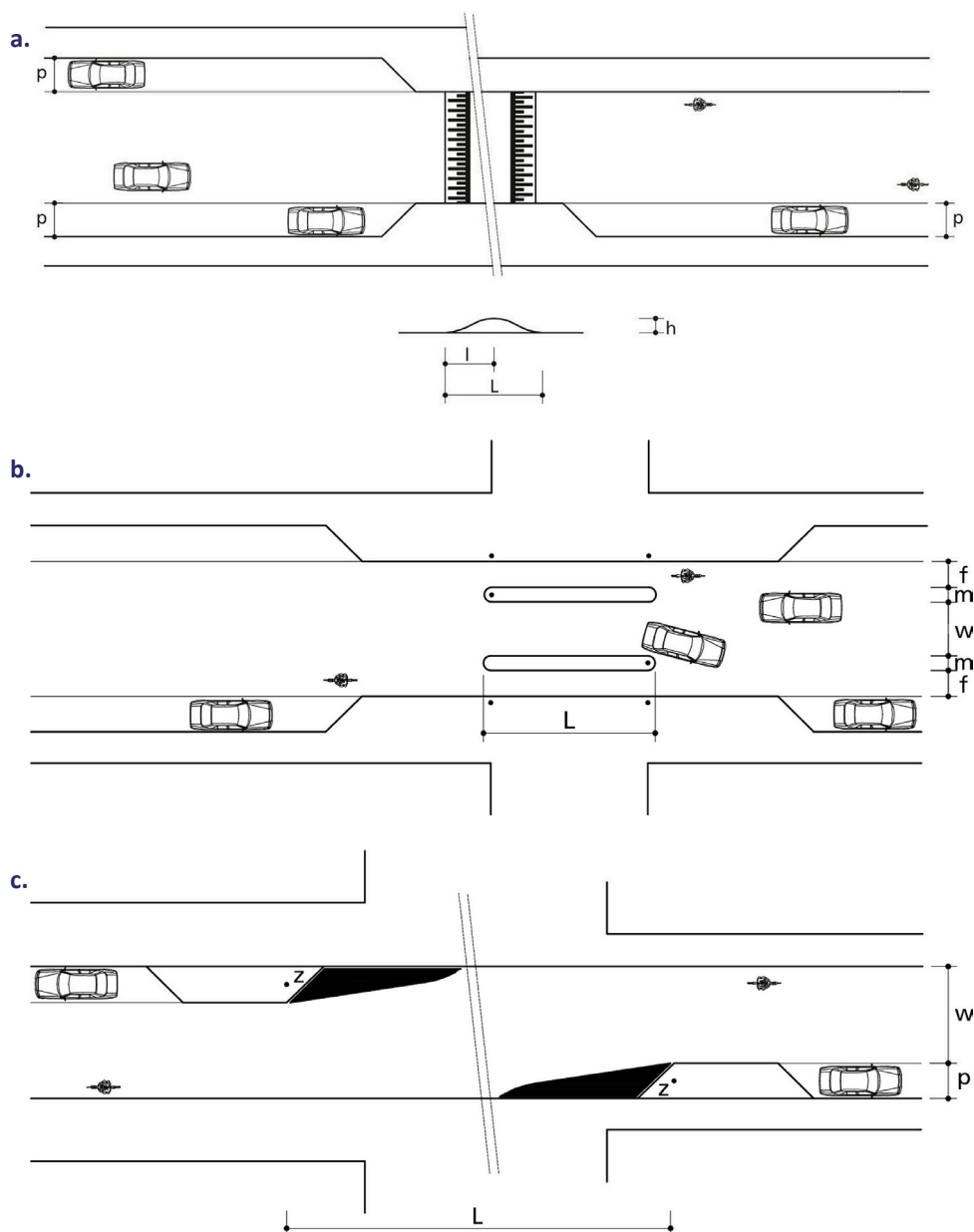
Afbeelding 5.3. Snelheidsremmers op erftoegangswegen binnen de bebouwde kom volgens ASVV 11.2.21, 11.2.24, 11.2.25 (CROW, 2021)
