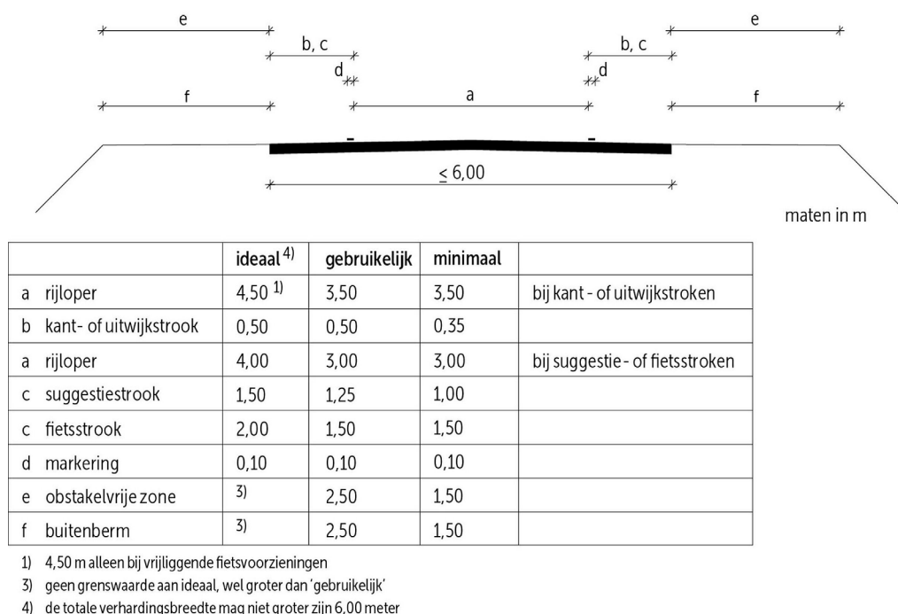
Afbeelding 5.9. Dwarsprofiel van erftoegangswegen buiten de bebouwde kom—Type 1 (CROW, 2013a)
