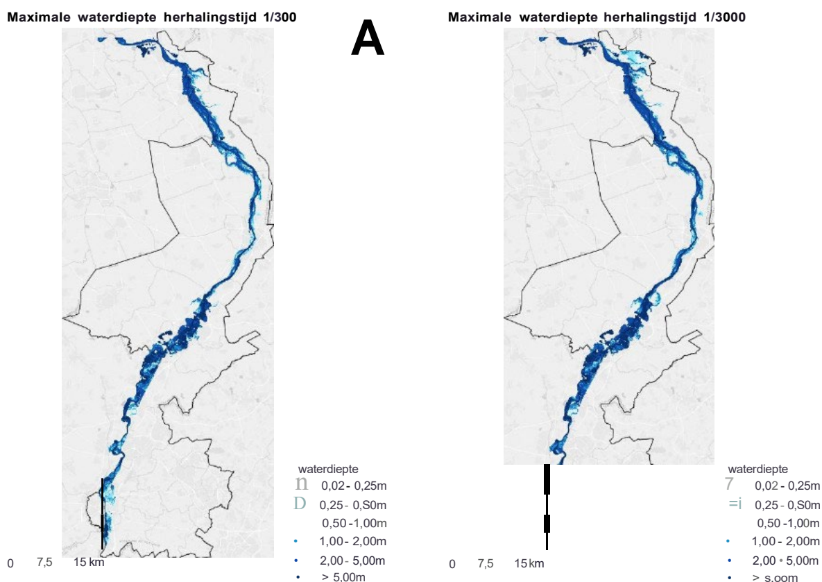
Figuur 5.5 Maximale waterdieptekaart Limburg. Links de maximale waterdiepte voor een afvoer met herhalingstijd 11300 jaar; rechts 113000 jaar. Kaartresolutie is 5x5m.
