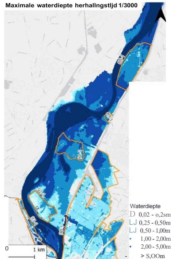
Figuur 5.6 Maximale waterdiepte kaart Limburg ingezoomd. Links de maximale waterdiepte voor een afvoer met herhalingstijd 11300 jaar; rechts 113000 jaar Kaartresolutie is 5x5m.
