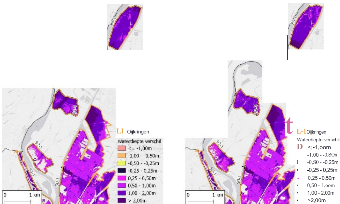
Figuur B4. Verschil in waterdiepte tussen nieuwe waterdieptekaarten en waqua-maas-j21_5-v1 waterdieptekaarten, als gebruikt in DPV. Een verschil groter dan nul (paars) betekent een grotere waterdiepte in de nieuwe waterdieptekaarten.
