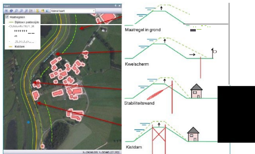
Figuur 3.4. Veronderstelde verdringingsreeks versterkingsmaatregelen in KOSWAT: van een gronddijk naar steeds zwaardere en duurdere constructieve maatregelen indien noodzakelijk door ruimtegebrek
