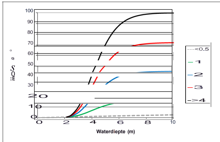
Figuur 2.4. De mortaliteit (in procenten) als functie van de waterdiepte voor locaties met een stijgsnelheid kleiner dan 0,5 m/uur, groter dan 4 m/uur en voor enkele tussenliggende waarden (stijgsnelheden van 1, 2 en 3 m/uur).
