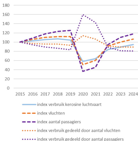
Figuur 3.33: Indices voor totaal energieverbruik, voor aantallen vluchten en passagiers en voor energieverbruik gedeeld door het aantal passagiers en gedeeld door het aantal vluchten
