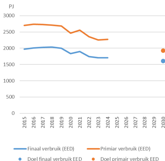
Figuur S.1: Totaal primair en totaal totaal energieverbruik conform de EED van 2015 tot en met 2024, de doelen uit Artikel 4 van de EED voor 2030 en de verbruiken uit de ramingen van de KEV 2025 in PJ
