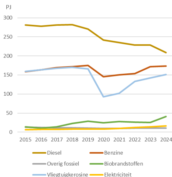
Figuur S.6: Finaal energieverbruik in de sector mobiliteit verdeeld naar energiedragers
