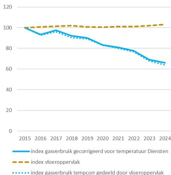
Figuur 3.23: Indices voor het voor temperatuur gecorrigeerd gasverbruik in de klimaatkkoordsector diensten, voor het vloeroppervlak en voor het gasverbruik gedeeld door het vloeroppervlak
