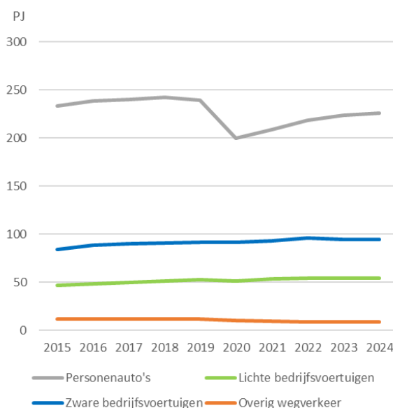
Figuur 3.28: Finaal energieverbruik personenauto's, vrachtwagens en lichte bedrijfsvoertuigen in PJ
