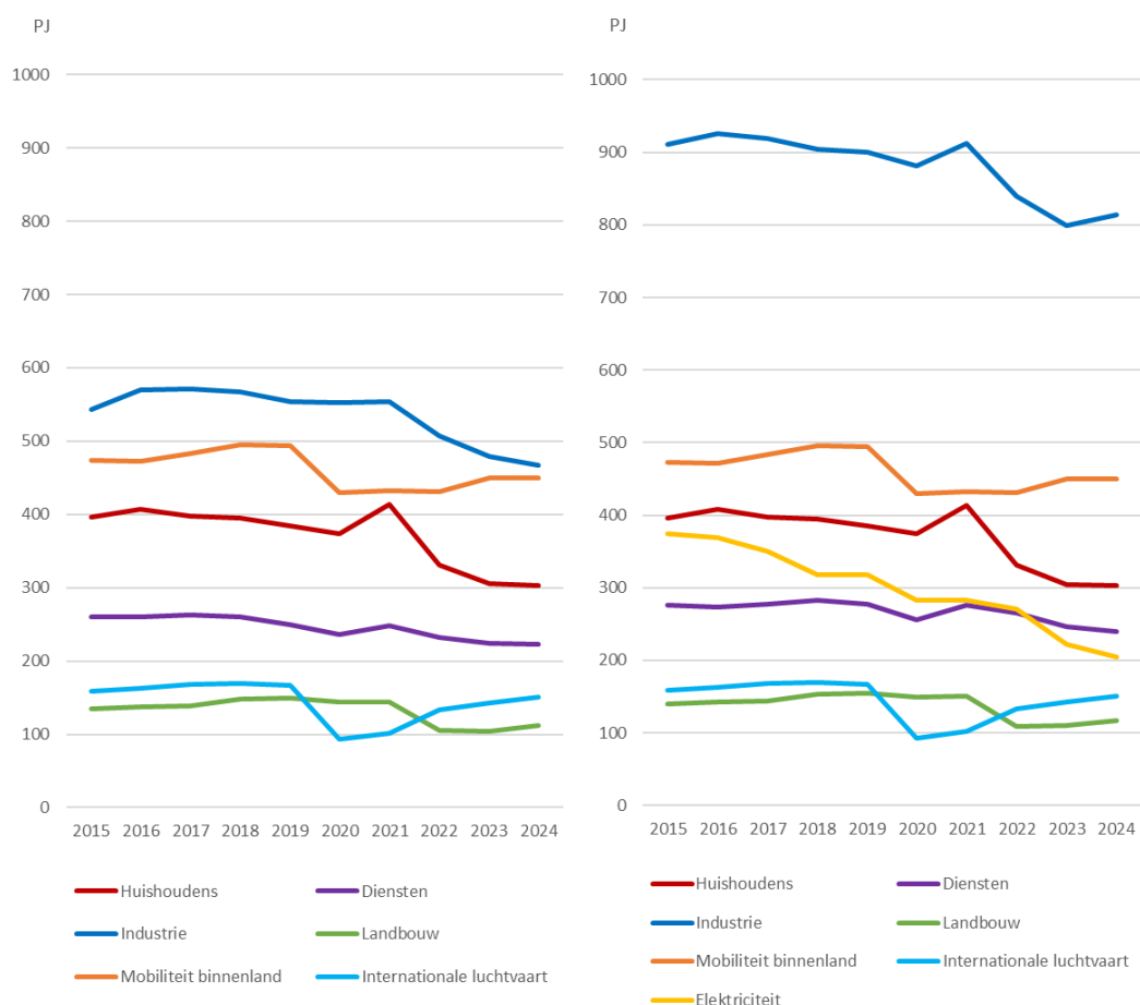
Figuur 3.2: Totaal finaal (links) en primair (rechts) energieverbruik per klimaatakkoordsector in PJ. Deze verbruiken zijn niet gecorrigeerd voor de buitentemperatuur
