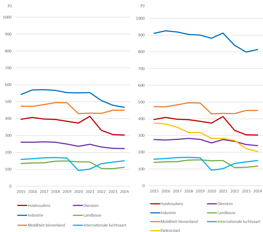
Figuur S.2: Totaal finaal (links) en primair (rechts) energieverbruik per klimaatakkoordsector in PJ. Deze verbruiken zijn niet gecorrigeerd voor de buitentemperatuur.
