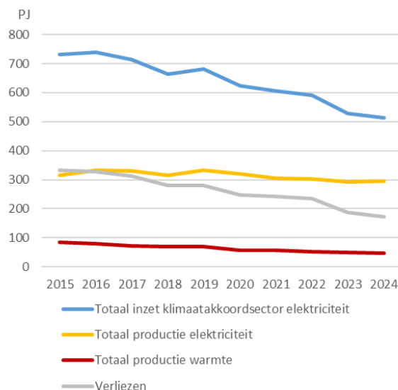
Figuur 3.6: Energie-inzet, productie van elektriciteit en warmte en verliezen in de klimaatkkoordsector elektriciteit in PJ
