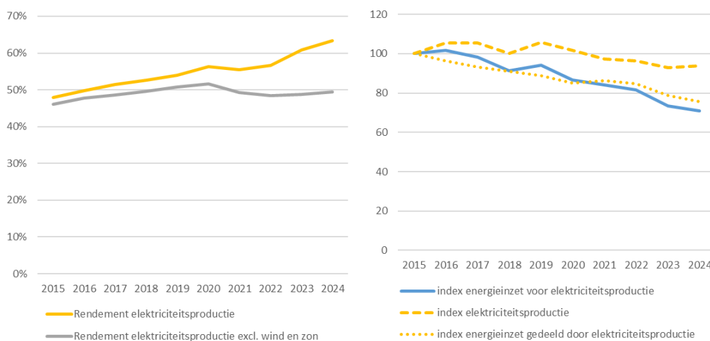
Figuur 3.7: Het rendement van de elektriciteitsopwekking in de klimaatkkoordsector elektriciteit (links) en indices voor de energie-inzet, voor de elektriciteitsproductie en voor de inzet gedeeld door de elektriciteitsproductie (rechts)
