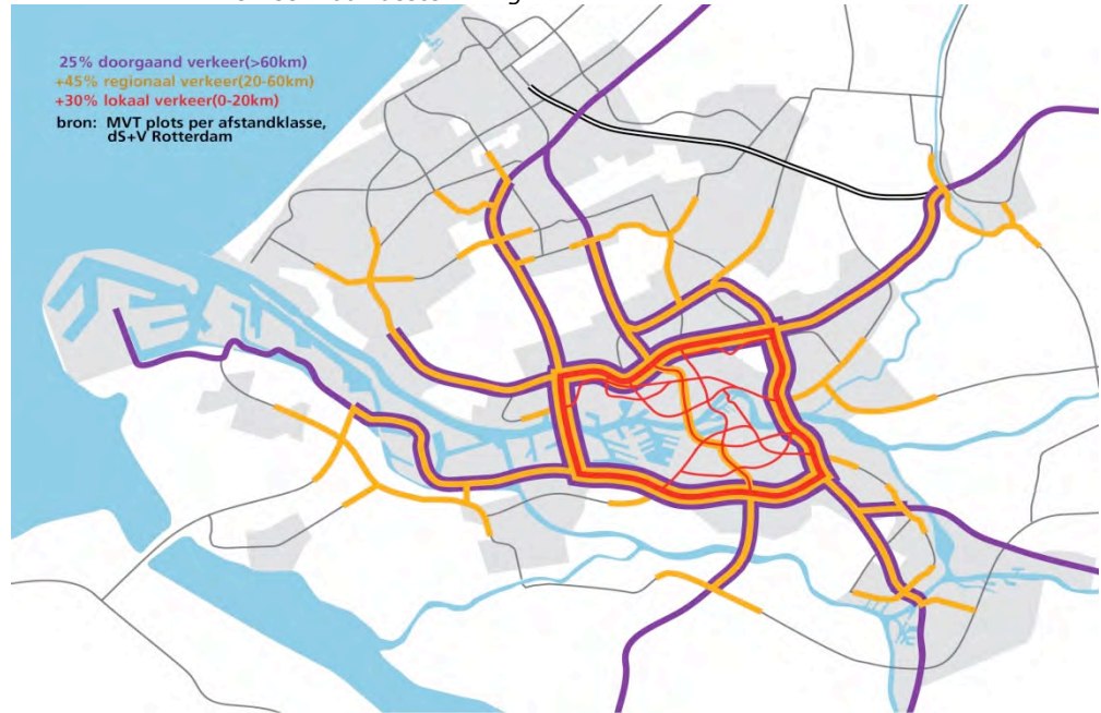
Afbeelding 4: verkeersplot van het regionale wegennet, inclusief een verdeling van het verkeer naar bestemming.
