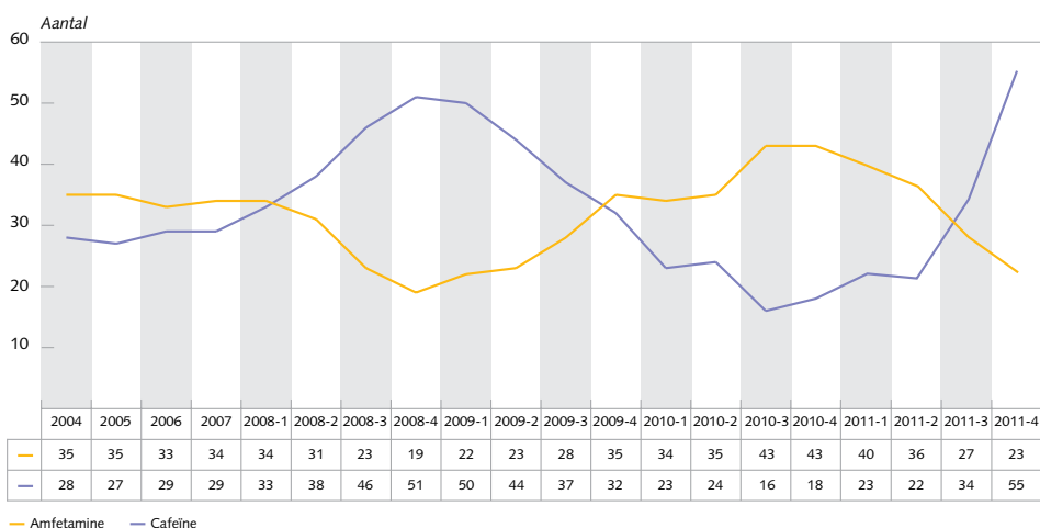
Figuur 5.9 Gehalte amfetamine en cafeïne in speedpoeders, vanaf 2004
