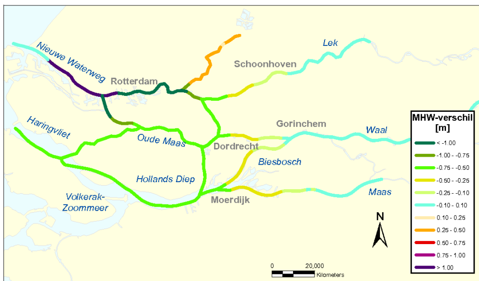
Figuur B4.3: MHW- effect ten opzichte van het huidig Beheer bij uitvoering van variant 'Afsluiten van Nieuwe en Oude Maas met inzet van Volkerak-Zoommeer + Oosterschelde en installatie van gemalen'; zichtjaar 2100; klimaatscenario W/W+ (HKV, 2015a).
