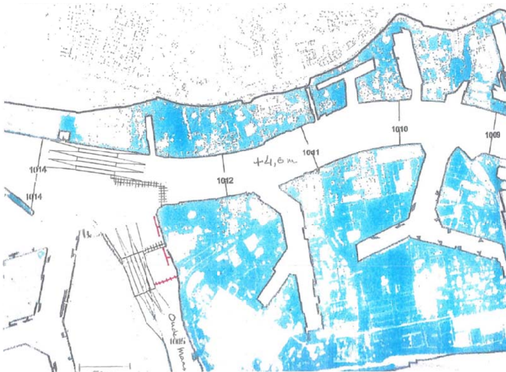
Fig. B7.1: Alternatief voor Plan Sluizen bij Vlaardingen. In blauw buitendijkse gebieden die achter de sluizen komen te liggen
