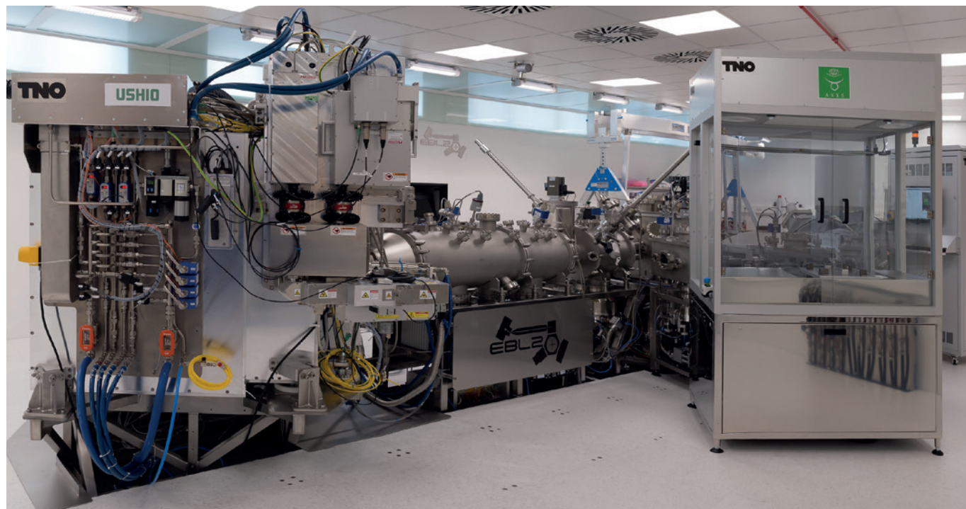
Extreem Ultra Violet (EUV) belichtings- en analysefaciliteit EBL-2 (TNO en USHIO)
