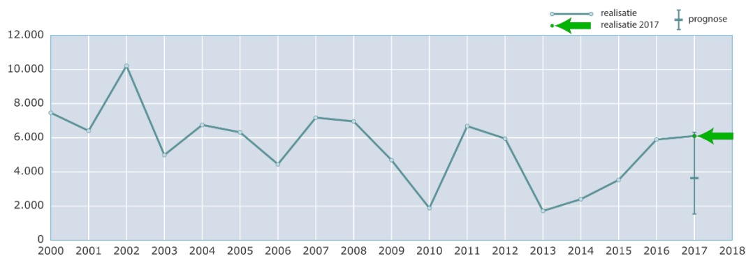
Figuur 6.3 Aantal woningen met een geluidbelasting van 48 dB(A) L_{night} of meer
