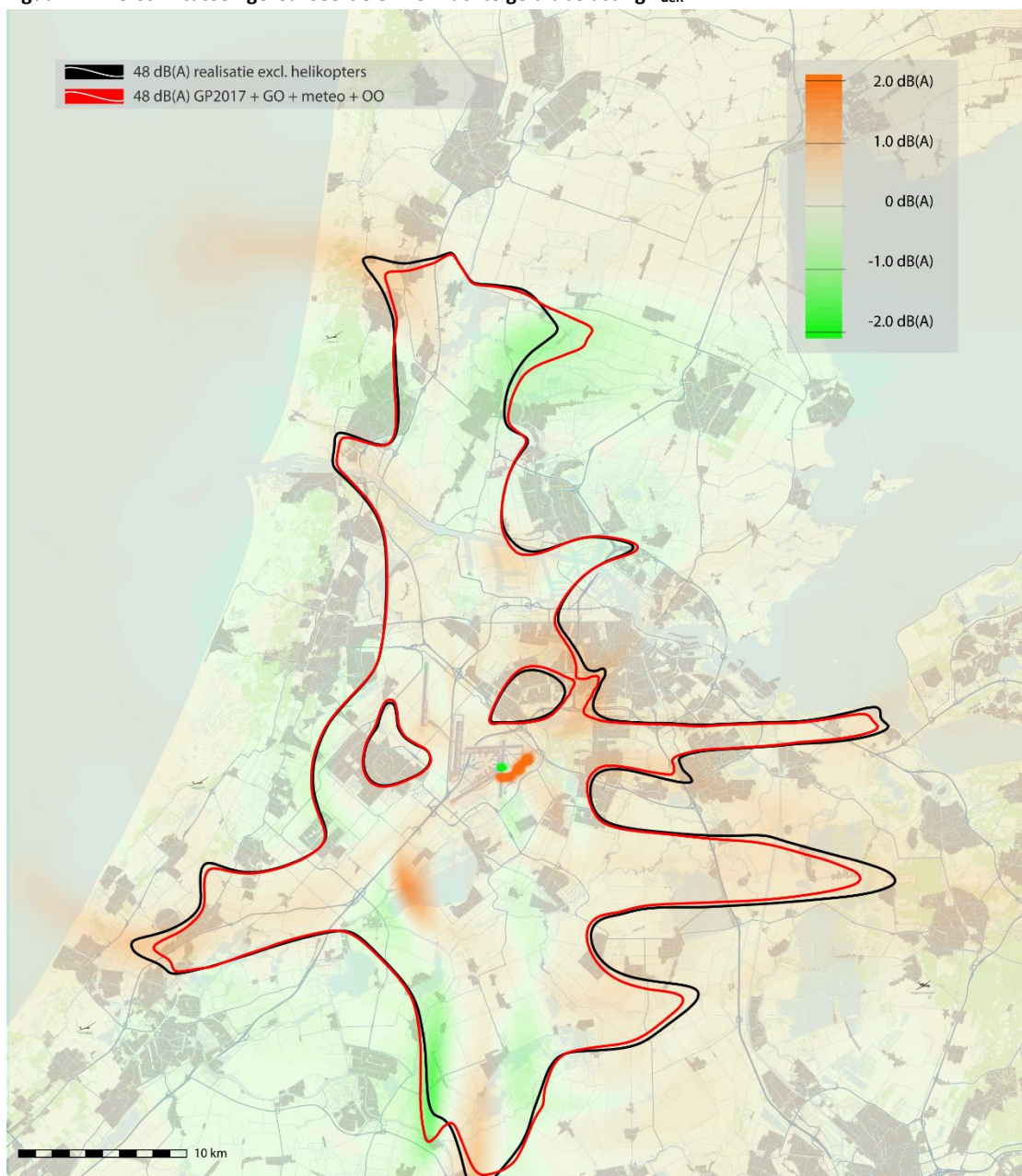
Figuur A.1 Verskil tussen gerealiseerde en verwachte geluidbelasting L_{den}
