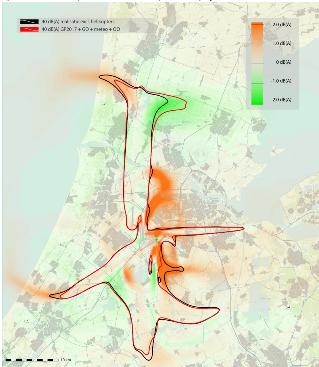
Figuur A.2 Verschil tussen gerealiseerde en verwachte geluidbelasting L_{night}
