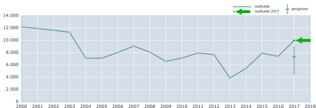
Figuur 6.2 Aantal ernstig gehinderden met een geluidbelasting van 48 dB(A) L_{den} of meer
