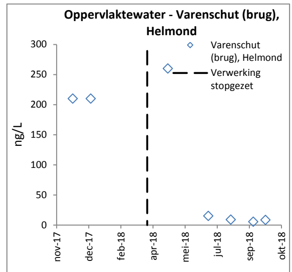
Figuur 28 Gehalten aan GenX-stoffen in openbaar oppervlaktewater nabij de kruising van de brug met Varenschut (Helmond), in de nabijheid van Custom Powders in Helmond. De verticale stippellijn geeft aan op welk moment Custom Powders is gestopt met werkzaamheden voor Chemours. Na deze datum lijken de gehalten te dalen.
