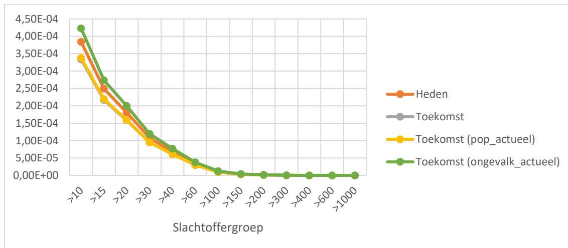
Figuur 4 FN-curve heden versus toekomst, toekomst (populatiebestand heden), toekomst (ongevalskansen heden) en toekomst (populatiebestand en ongevalskansen heden).
