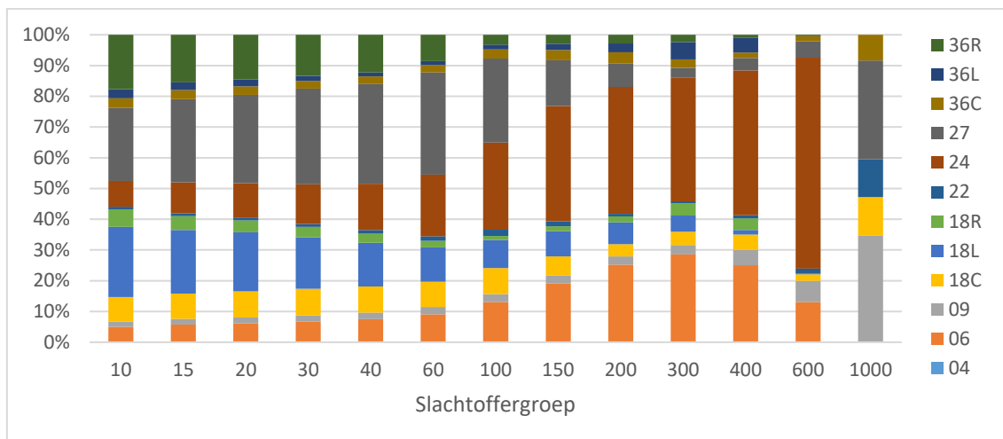
Figuur 15 Percentage van totale groepsrisico per baan per slachtoffergroep voor de toekomst.
