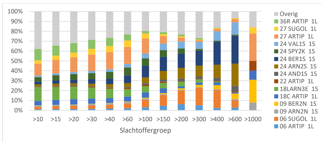
Figuur 10 Percentage van totale groepsrisico per route voor het verleden met het actuele populatiebestand.
