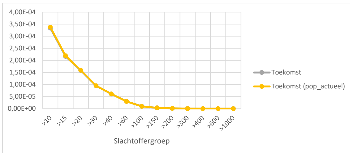
Figuur 18 FN-curve voor de toekomst met toekomstig en actueel populatiebestand.
