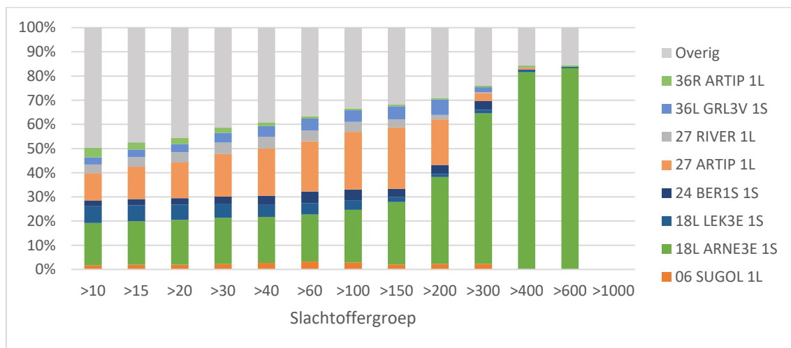
Figuur 9 Percentage van totale groepsrisico per route voor het verleden.
