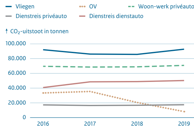
Figuur 9.6: Uitstoot per jaar naar vervoerssoort in ton CO 2 .
