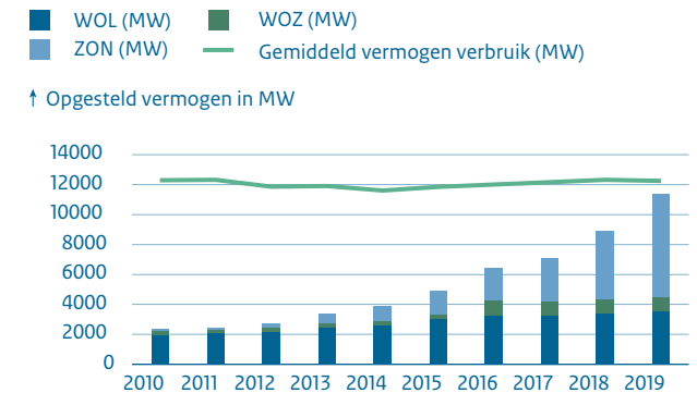
Figuur 1.13: Verhouding totaal elektriciteitsverbruik en productie Zon, WoL en WOZ. Bron: CBS (2020)
