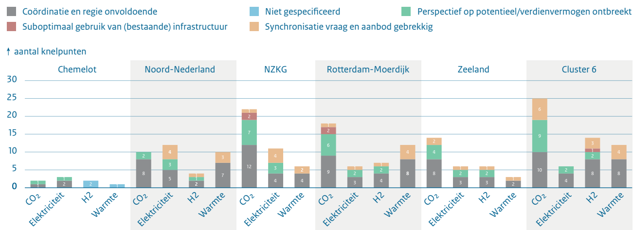
Figuur 2.1: Knelpunten infrastructuur per techniek, naar type knelpunt en per industrieccluster.
