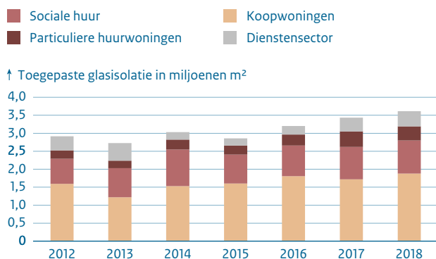
Figuur 3.13: In bestaande bouw toegepaste glasisolatie. Bron: RVO (2019)
