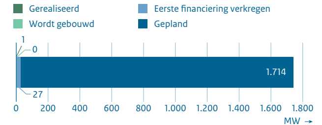
Figuur 1.9: Gepland vermogen in waterstofprojecten uit elektrolyse in 2019 5 . Bron: RVO (2020); TKI Nieuw Gas (2020); Gasunie (2020)
