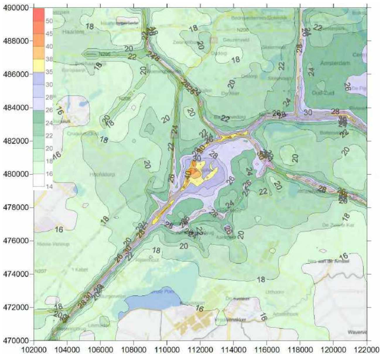
Figuur K.3: Contourplot (20x20 km) van de jaargemiddelde concentratie NO 2 (in µg/m 3 ) scenario 450k_NNHS zichtjaar 2020
