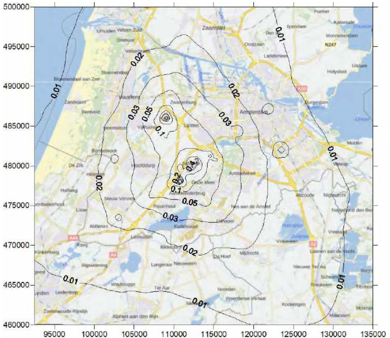
Figuur K.21: Contourplot (42,5x40 km) van de jaargemiddelde concentratie PM_{10} (in \mu\text{g}/\text{m}^3 ): de bijdrage van de luchtvaartbronnen en grondbronnen scenario 450k_HS zichtjaar 2020
