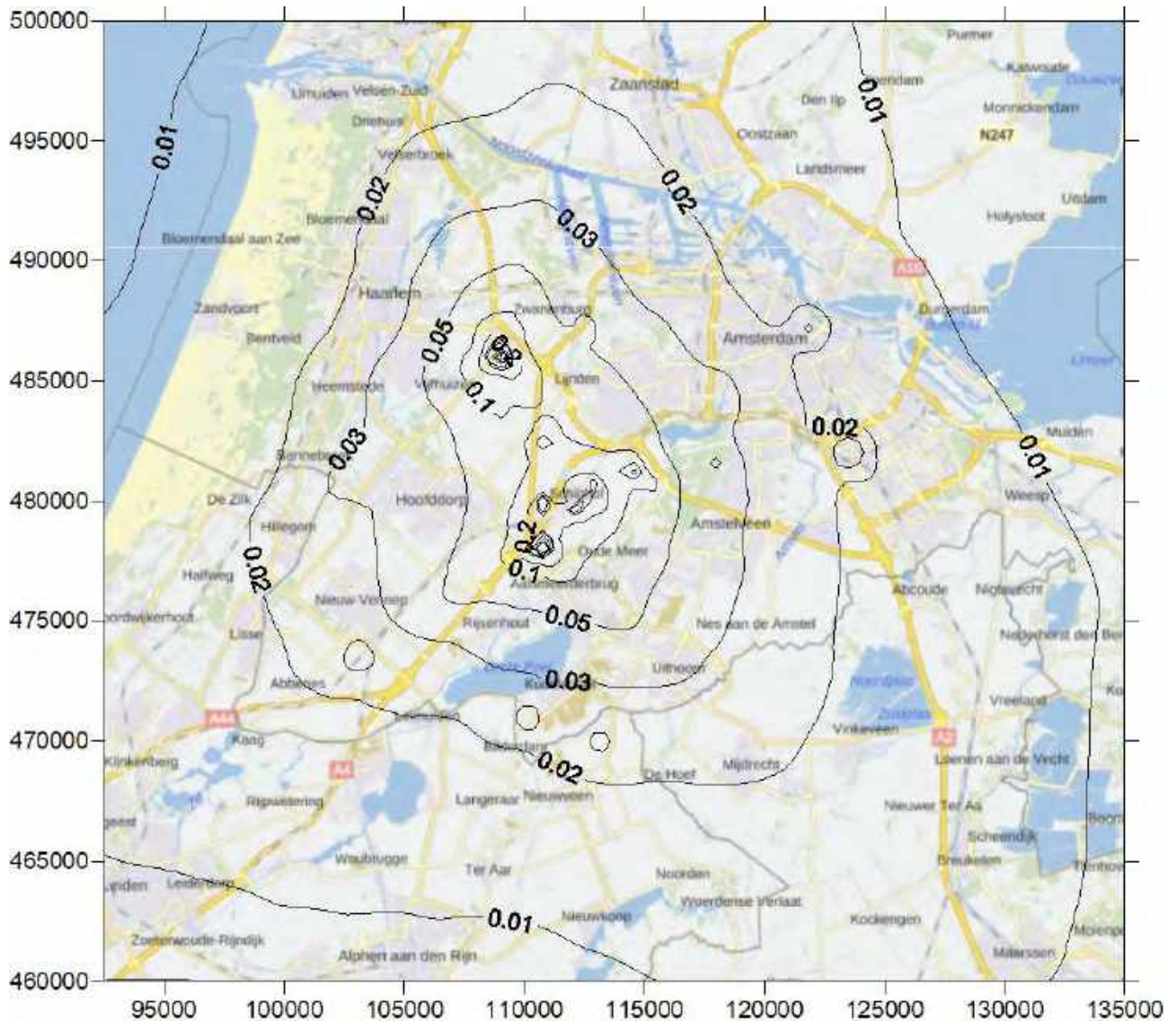
Figuur K.24: Contourplot (42,5x40 km) van de jaargemiddelde concentratie PM 10 (in µg/m 3 ): de bijdrage van de luchtvaartbronnen en grondbronnen scenario 500k_NNHS zichtjaar 2025
