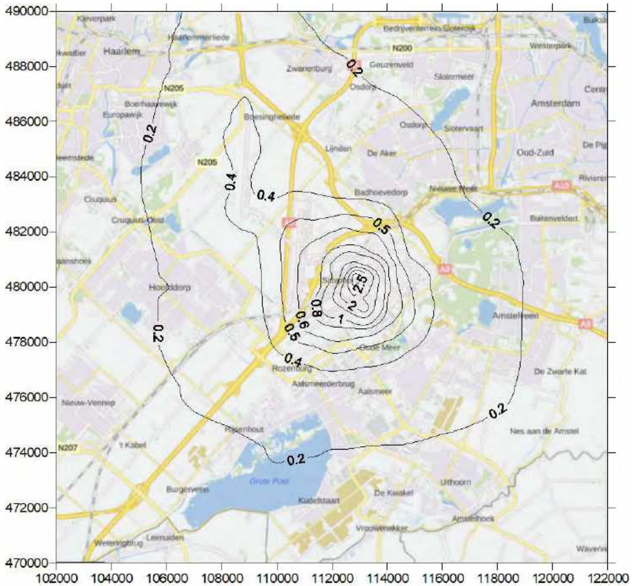
Figuur K.44: Contourplot (20 x 20 km) van de 98 percentiel VOS scenario 450k_HS (2015) in ouE/m^3
