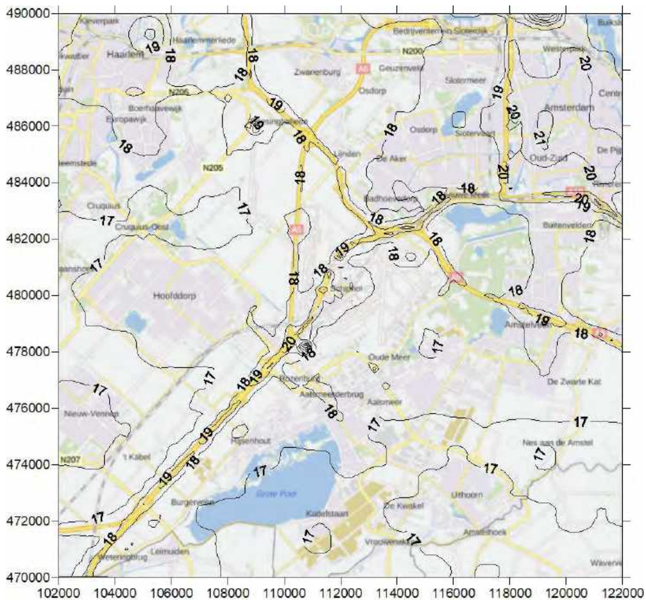
Figuur K.17: Contourplot (20x20 km) van de jaargemiddelde concentratie PM 10 (in µg/m 3 ) scenario 500k_NNHS zichtjaar 2020
