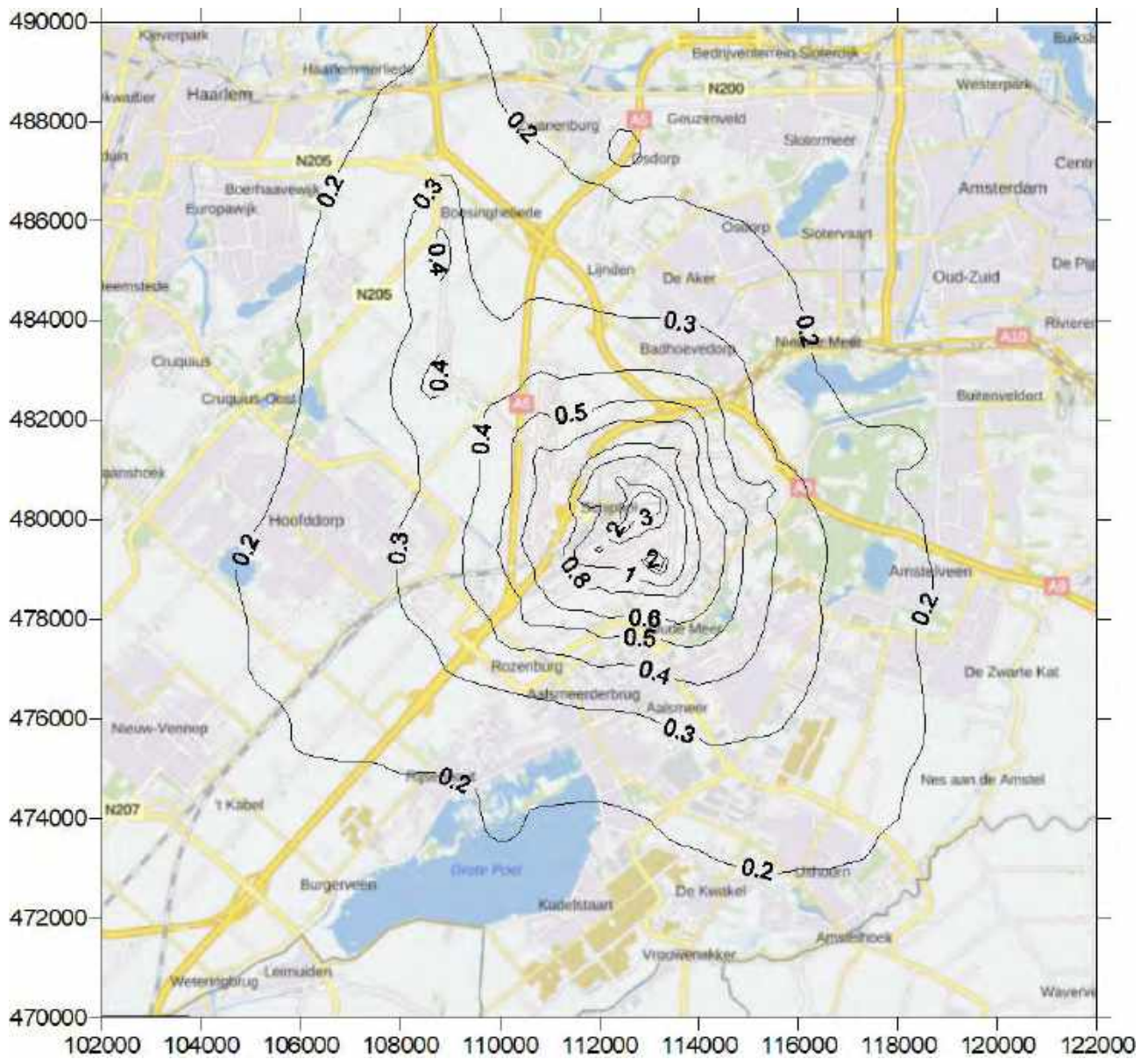
Figuur K.47: Contourplot (20 x 20 km) van de 98 percentiel VOS scenario 500k_NNHS (2020) in ouE/m^3
