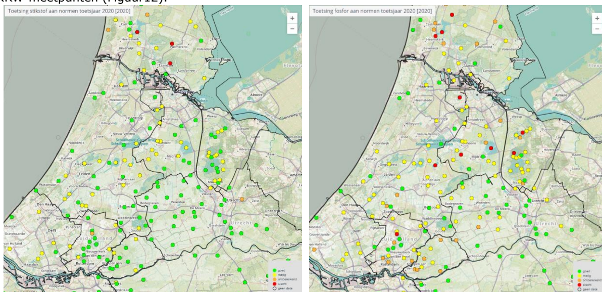
Figuur 12. Toestandsbeoordeling voor 2020 van de N-concentraties (links) en P-concentraties (rechts) op de KRW-meetpunten in west Nederland (Bron: KRW-Nutrend).
