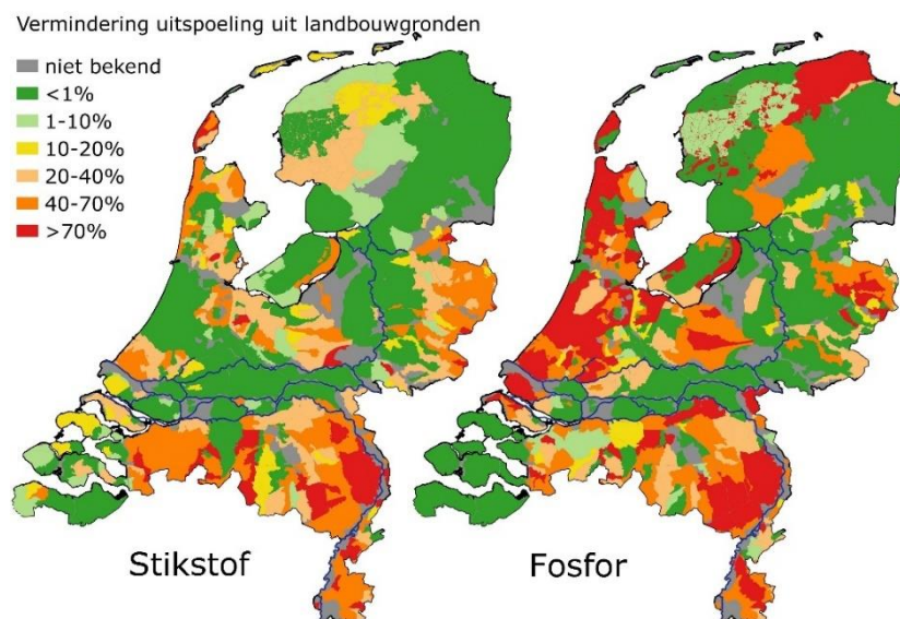
Figuur 3. Benodigde vermindering van de N- en P-uitspoeling uit landbouwgronden om aan de doelen van de Kaderrichtlijn Water te kunnen voldoen (bron: Groenendijk & Van Boekel, WaterMatter 2017).
