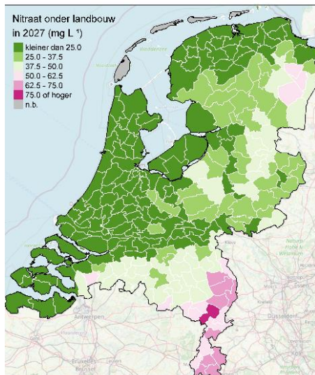
Figuur 1. Berekende nitraatconcentratie onder landbouwgrond in 2027 bij een maximale inzet van DAW-maatregelen (scenario 'maximaal' in Nationale Analyse) en benadering van een hoger aandeel rustgewassen in het bouwplan van akker- en tuinbouwbedrijven.
