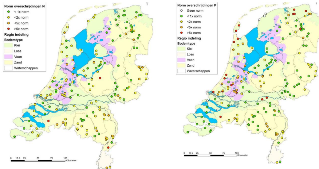
Figuur 2. Mate van overschrijding van N- en P-concentraties in het Meetnet Nutriënten Landbouw Specifiek Oppervlaktewater (MNLISO) in de periode 2015 – 2018 ten opzichte van doelen voor KRW-waterlichamen 2 (Bron: Buijs et al, 2020; Deltares-rapport 11203728-005-BGS-0002).
