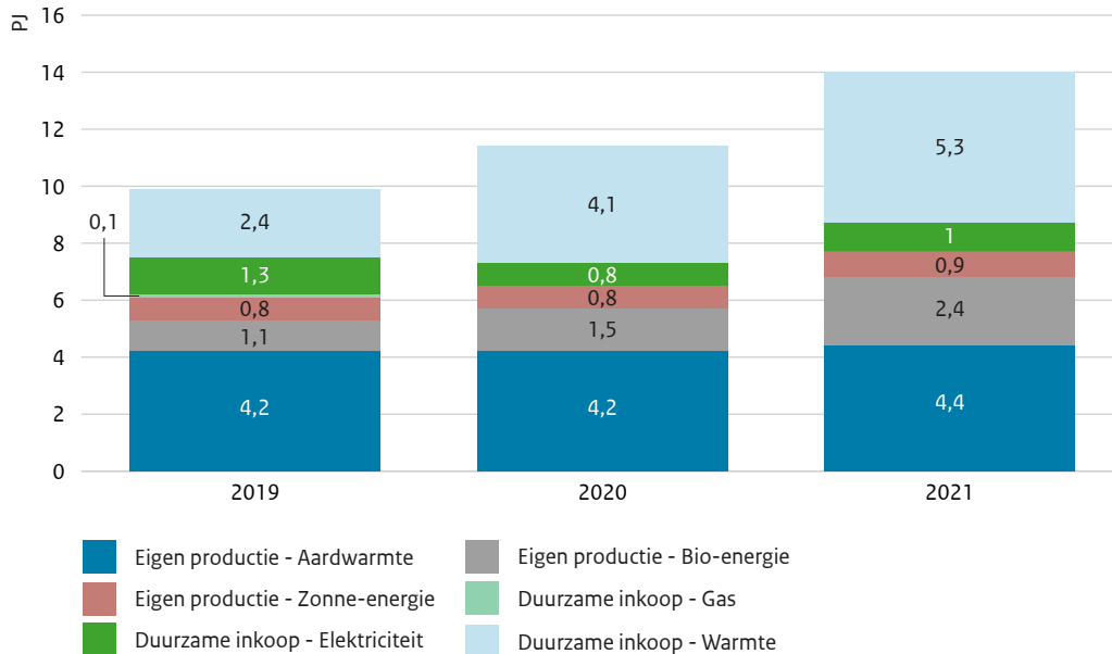
Figuur 25. Verbruik duurzame energie glastuinbouwsector. Data voor 2022 komen pas na publicatie van deze nota beschikbaar.
