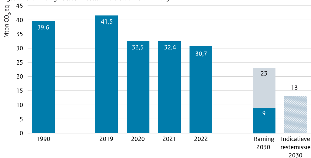
Figuur 2. Ontwikkeling uitstoot in de sector Elektriciteit. Bron: KEV 2023
