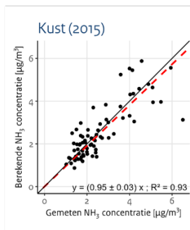
Figuur 11 Scatterplots van de ruimtelijk gekalibreerde berekende versus de gemeten ammoniakconcentraties waarbij de oude zee-emissies zijn meegenomen (links), waarbij de oude zee-emissies niet zijn meegenomen (midden) en waarbij de drie aanpassingen zijn meegenomen (rechts).
