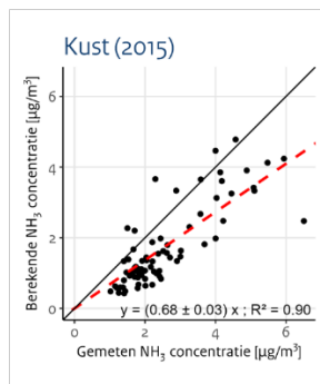
Figuur 10 Scatterplots van de ongekalibreerde berekende versus de gemeten ammoniakconcentraties waarbij de oude zee-emissies zijn meegenomen (links), waarbij de oude zee-emissies niet zijn meegenomen (midden) en waarbij de drie aanpassingen zijn meegenomen (rechts).
