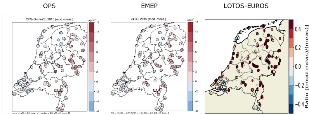
Figuur 9 Verschil tussen berekende en gemeten ammoniakconcentraties in 2015 in Nederland voor OPS (RIVM), EMEP (RIVM) en LOTOS-EUROS (TNO). N.B.: de berekeningen voor LOTOS-EUROS zijn relatief ten opzichte van de metingen, maar dit maakt voor het beeld niet uit. Dit verklaart waarom de schaalverdeling anders is.
