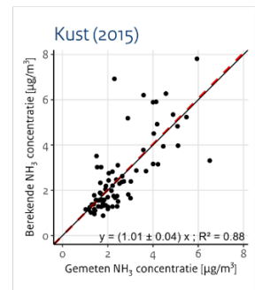
Figuur 11 Scatterplots van de ruimtelijk gekalibreerde berekende versus de gemeten ammoniakconcentraties waarbij de oude zee-emissies zijn meegenomen (links), waarbij de oude zee-emissies niet zijn meegenomen (midden) en waarbij de drie aanpassingen zijn meegenomen (rechts).
