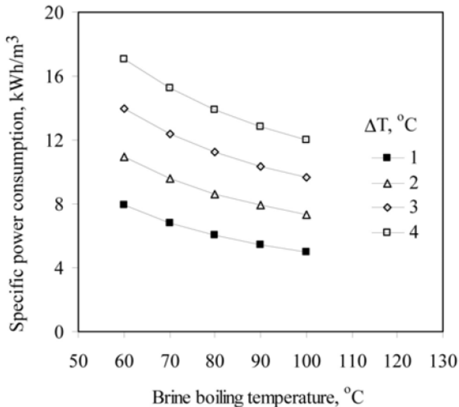
Figuur 4. Benodigd vermogen in single effect MVC als functie van temperatuursverschil over de warmtewisselaar bij verschillende brijn kooktemperaturen. Overgenomen uit Desalination 2006 190 1–15.
