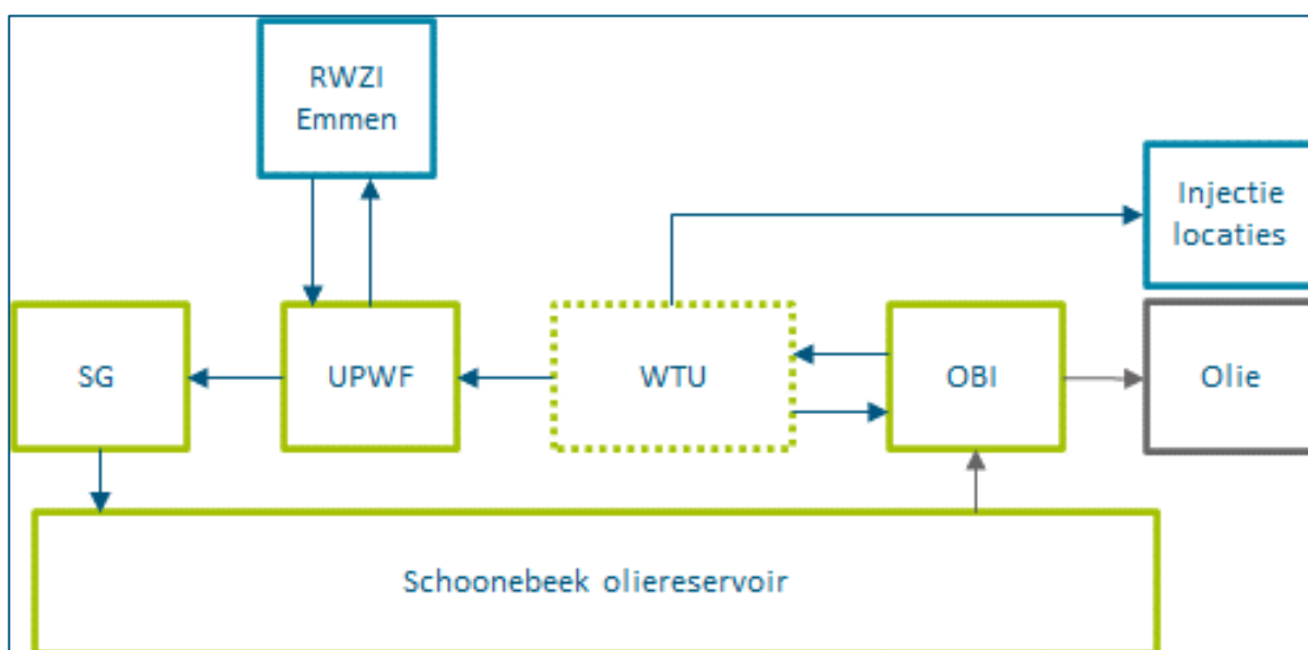
Figuur 7-1. Voorgesteld circulair concept (toelichting afkortingen: RWZI: rioolwaterzuiveringsinstallatie, SG: stoomgeneratie, UPWF: ultrapuure waterfabriek, WTU: voorbehandelingsinstallatie, OBI: olie-behandelingsinstallatie)
