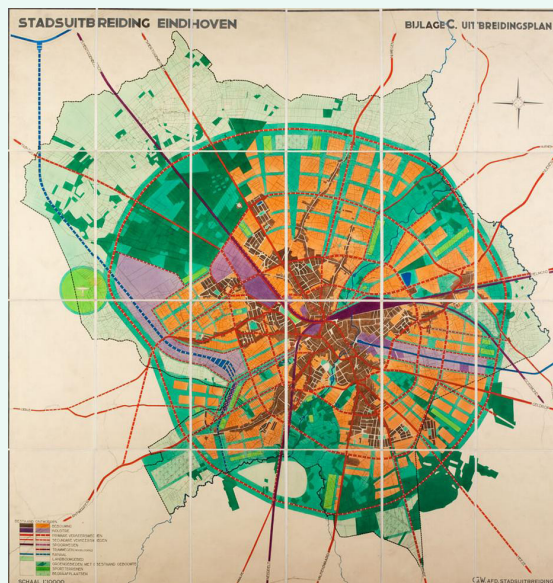
Uitbreidingsplan Eindhoven, 1930
