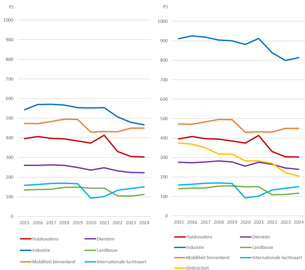
Figuur 3.2: Totaal finala (links) en primair (rechts) energieverbruik per klimaatakkoordsector in PJ. Deze verbruiken zijn niet gecorrigeerd voor de buitentemperatuur
