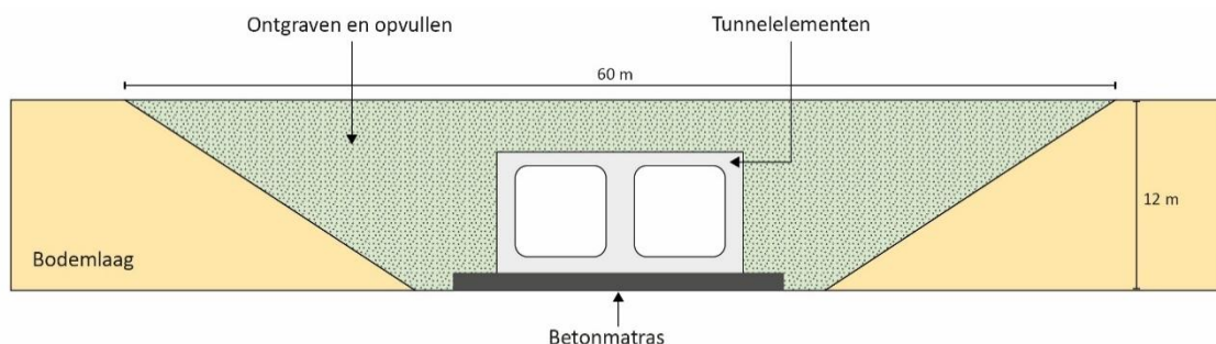
Figuur 5-12: Doorsnede afgezonken tunnel
