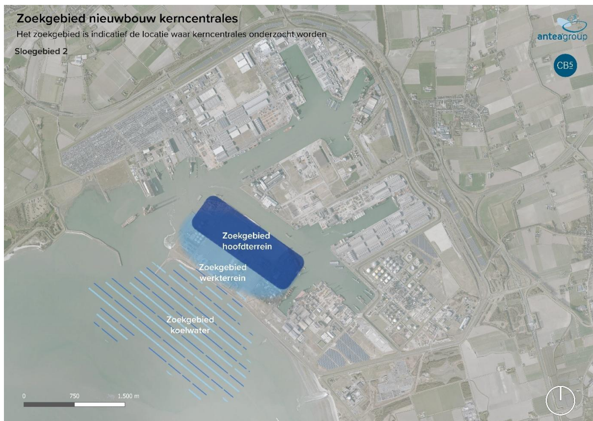
Figuur 4-8: Alternatief Sloegergebied 2
